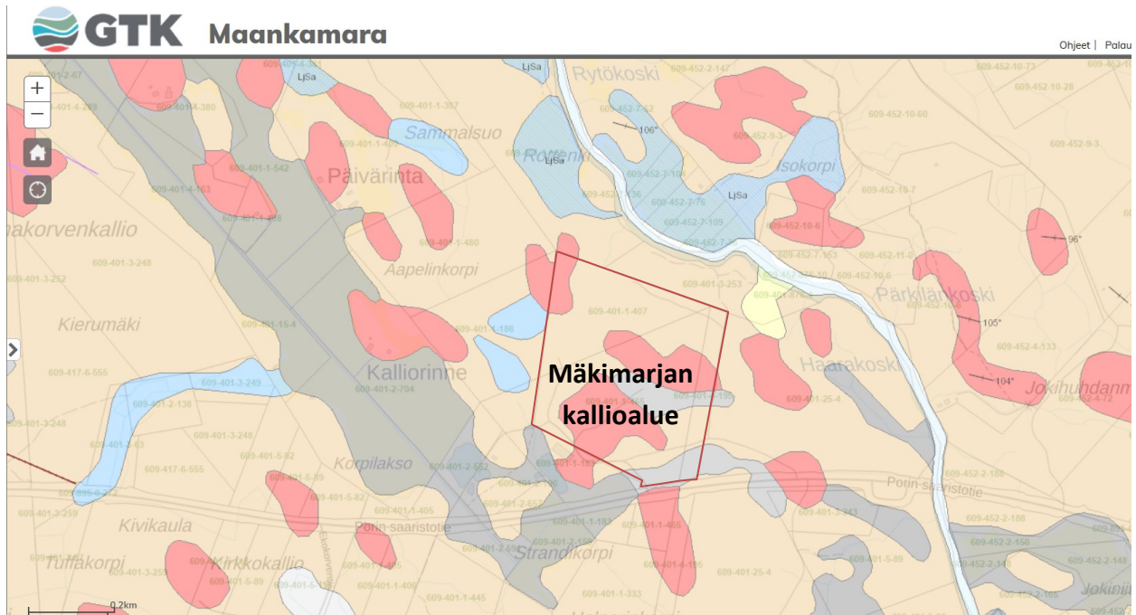
Kuva 1. Maaperäkarta. Ottamisalueen tilat on osoitettu rajauksena. Alueella pintamaalajit on poistettu. Niitä ovat olleet hiekkamoreeni (beige) ja saraturve (harmaa). Pohjamaalaji on kaikkialla kalliota. Länsipuolella on pienialaisia savikoita (sininen). Mittajana 0,2 km on kartan vasemmassa alakulmassa. Lähde: GTK, Maanmittauslaitos, Esri Finland. 2026.
