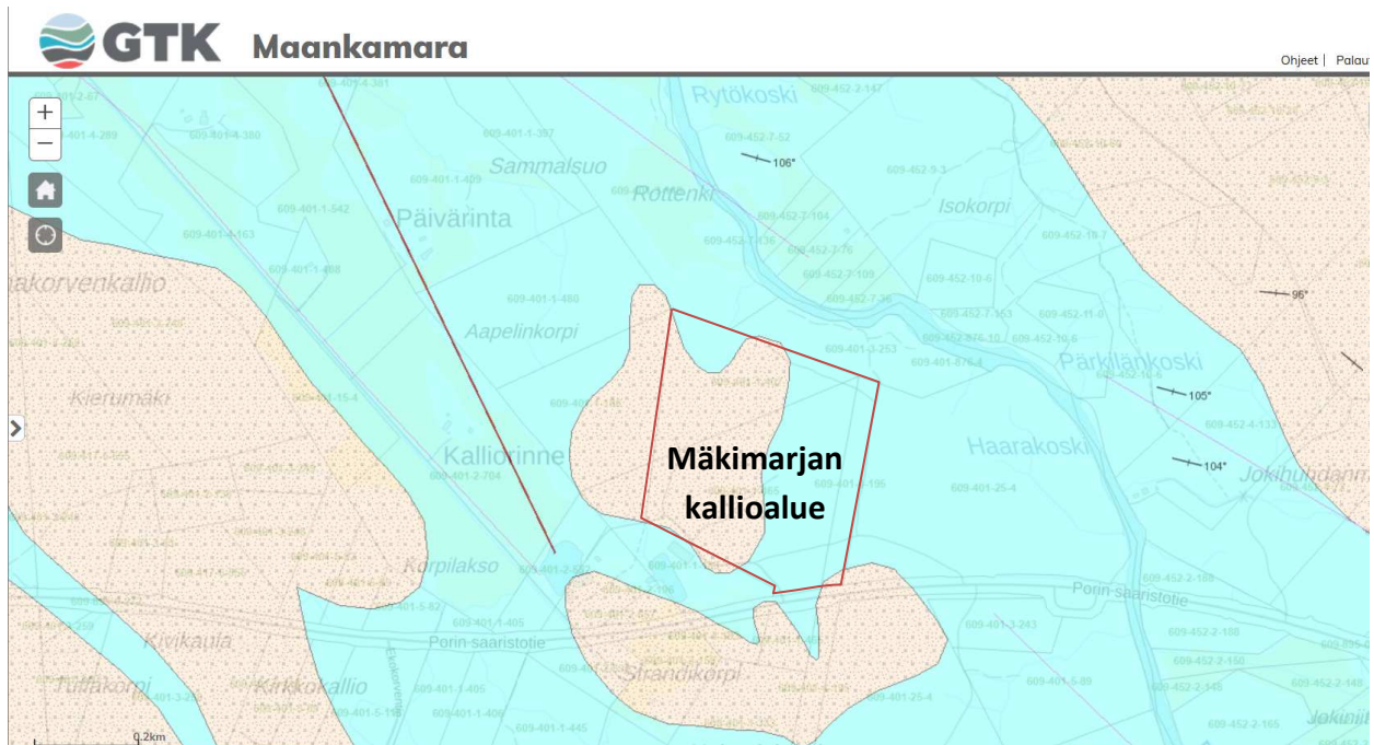
Kuva 2. Kallioperäkarta. Ottamisalueen tilat on osoitettu rajauksena. Ottamisalueen kallioperä koostuu sekä tonaliitista ja metagrauvakasta, kiilleliusketta ja kiillegneisiä. Viivalla esitetty diabaasijuoni. Uurteet 104...106 kulmassa. Mittajana 0,2 km on kartan vasemmassa alakulmassa. Lähde: GTK, Maanmittauslaitos, Esri Finland 2026.
